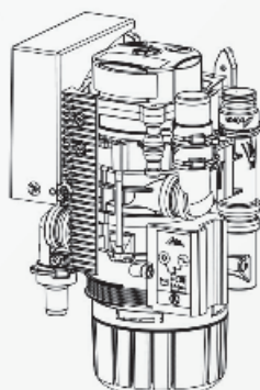
AMALGAM SEPARATOR
