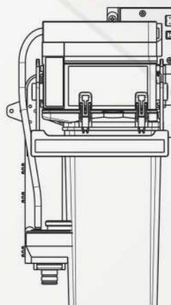
SEPARADOR AIRE/AGUA
