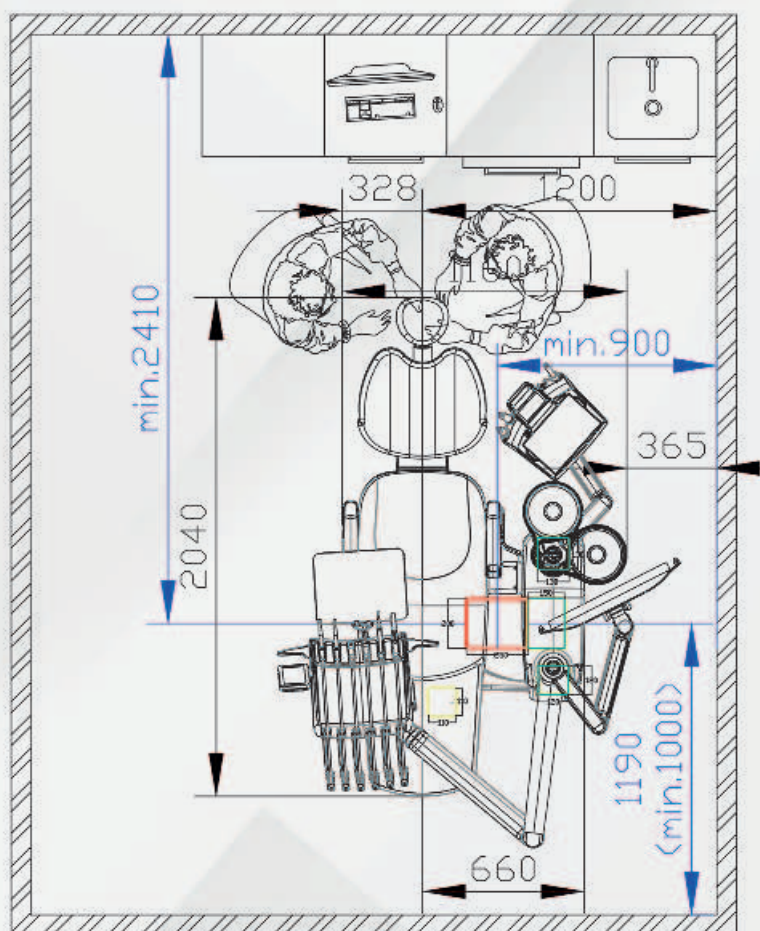
DIMENSIONS GLOBALES (Dimensions en millimètres)
