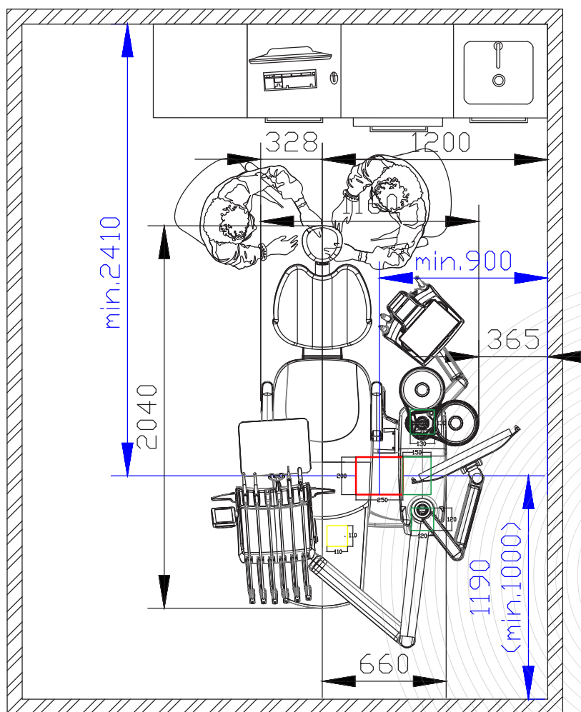
DIMENSIONI D'INGOMBRO (Misure in millimetri)
